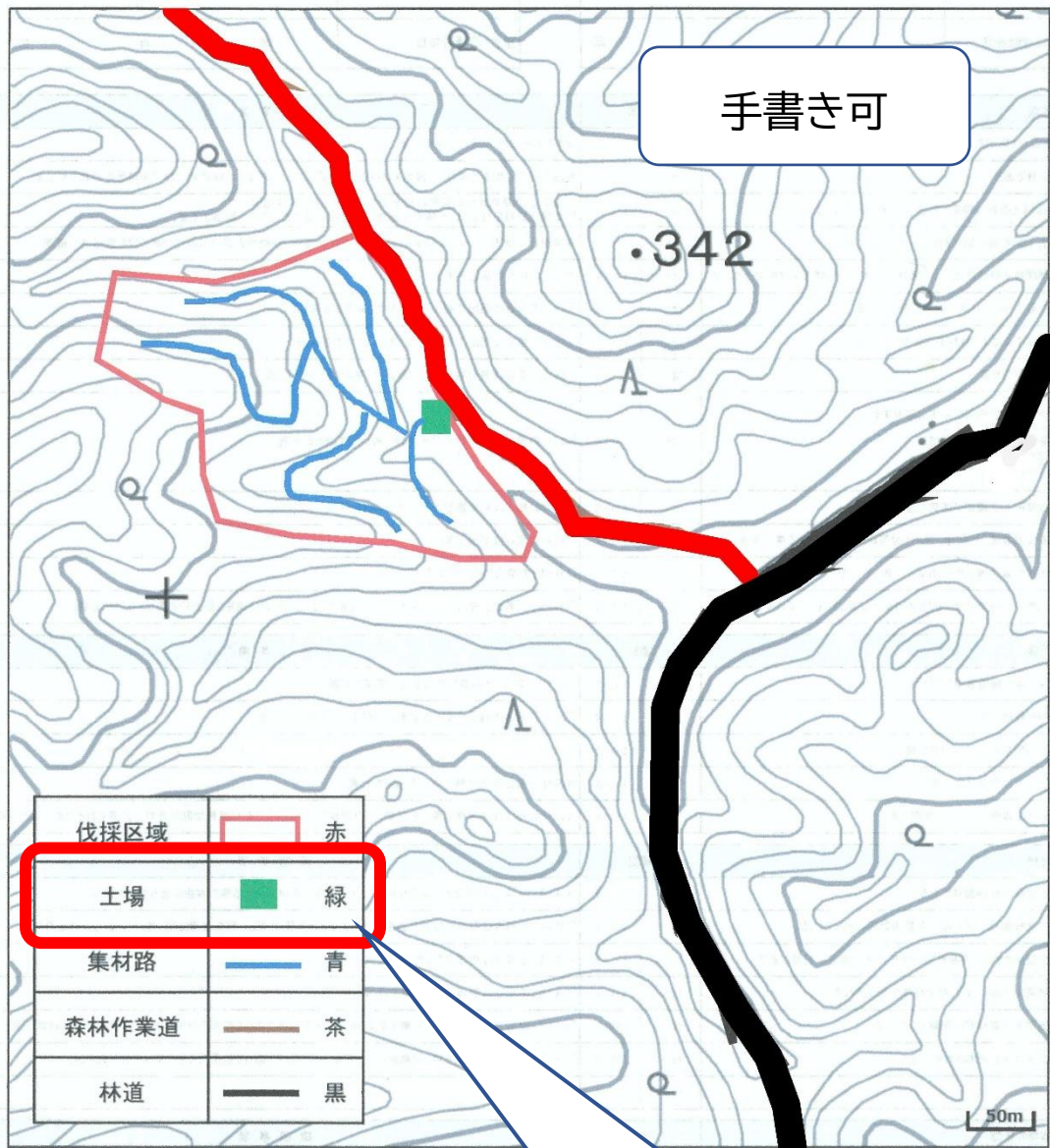
搬出計画図（例）
