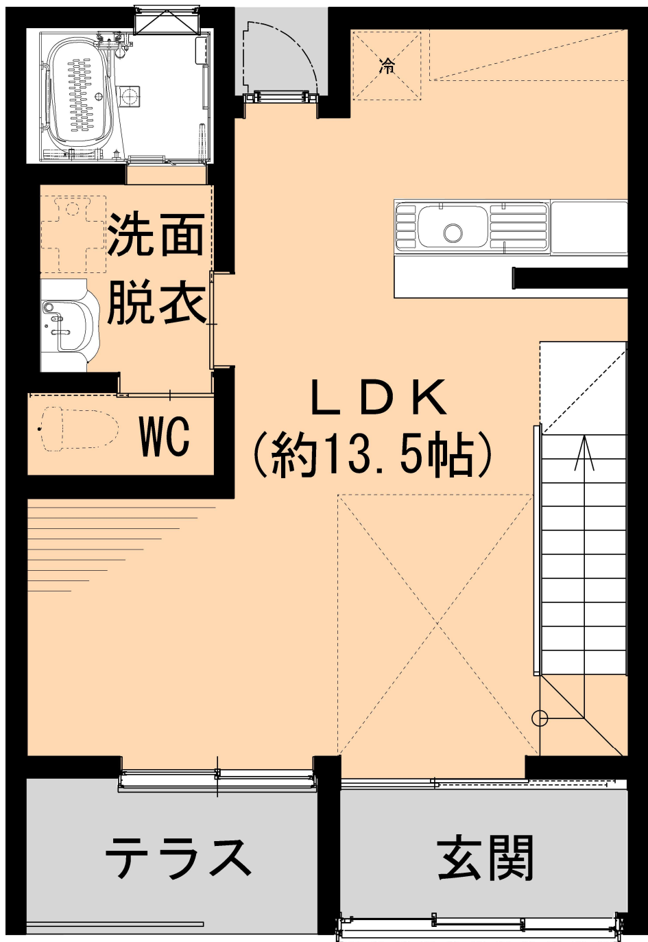
家族世帯向け住宅 1階
